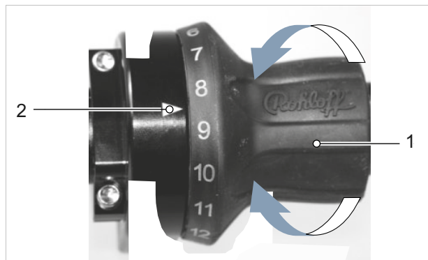
Illustration 174 : Poignée rotative ROHLOFF avec manette de vitesse (1) et affichage (2)
