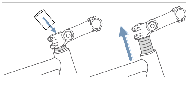
Illustration 115 : Relever la potence Ahead en montant une rondelle d'écartement
