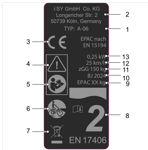
Illustration 2 : Exemple d'une plaque signalétique ZEG
