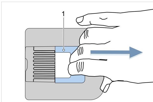
Illustration 178 : Tirer le verrou de pliage de la pédale (1) vers le bas
