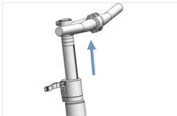
Illustration 113 : Tirer le guidon vers le haut, exemple d'un All Up
