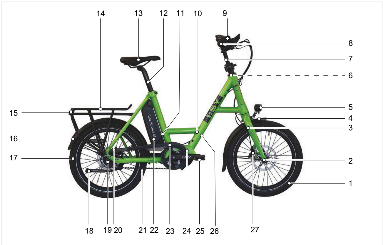
Illustration 4 : Vélo électrique vu de droite
