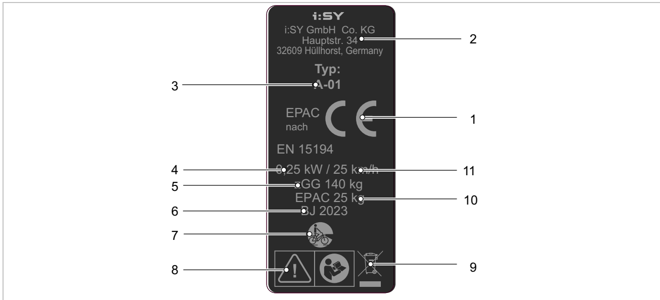
Illustration 3 : Exemple d'une plaque signalétique i:SY
