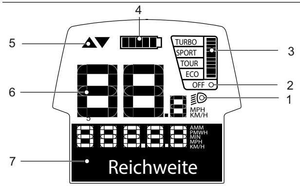
Figura 40: Vista general de la visualización del ordenador de a bordo
