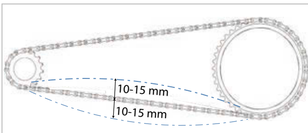
Figura 152: Comprobación de la tensión de la cadena
