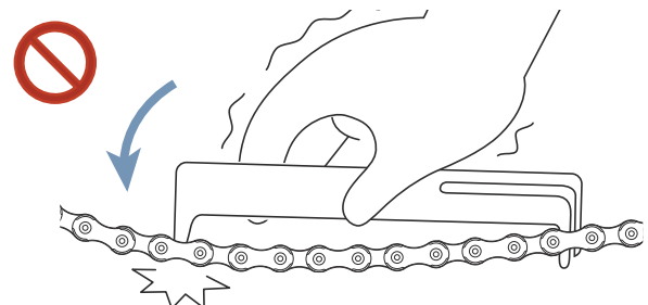
Figura 139: El calibre de medición cabe
