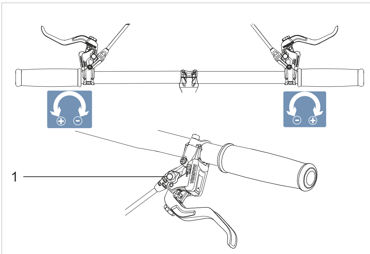
Figura 86: Utilización del botón giratorio (1) para el ajuste del punto de presión
