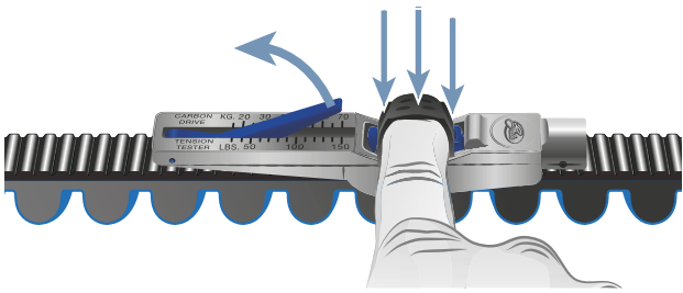
Figura 146: Presionar el calibre de comprobación hacia abajo
