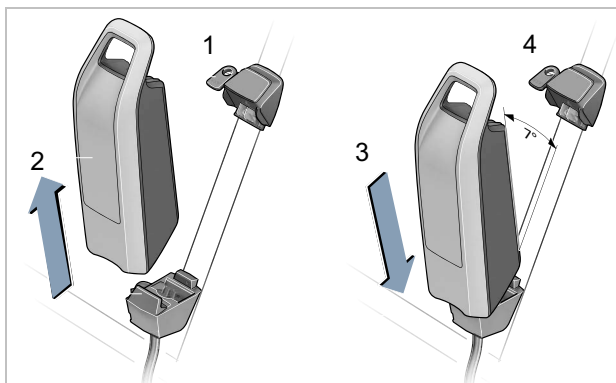
Figura 114: Extracción e inserción de la batería en el cuadro
