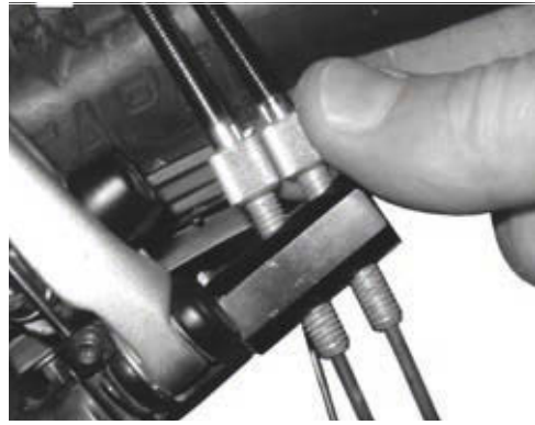
Figura 153: Las versiones de bujes ROHLOFF con activación de cambio interna tienen los dispositivos de ajuste de tensión en el contraapoyo de tensión
