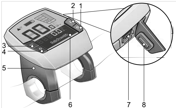
Figura 39: Estructura del ordenador de a bordo BOSCH Intuvia
