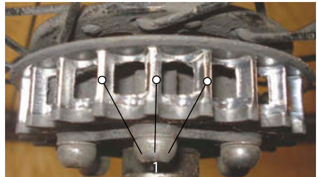
Figura 143: Fotografía de ejemplo de un perfil dentado desgastado
