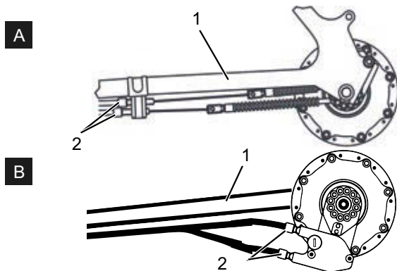
Figura 155: Casquillos de ajuste (2) en dos versiones alternativas (A y B) de un cambio de marchas accionado por cable de accionamiento, de dos cables en la vaina (1)
