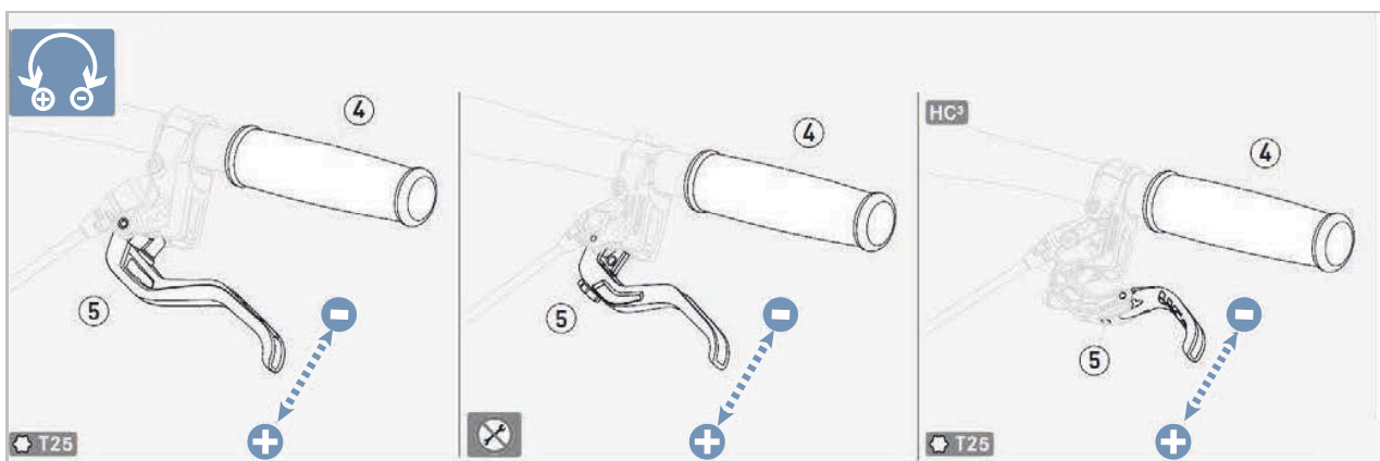
Figura 85: Ajuste del ancho de agarre del freno de mano con freno de disco MAGURA
