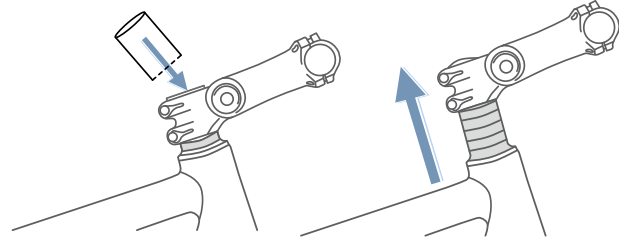
Figura 75: Aumento de la potencia Ahead mediante el montaje de anillos distanciadores (reductores)
