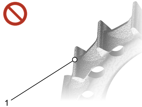
Figura 142: Perfil dentado desgastado
