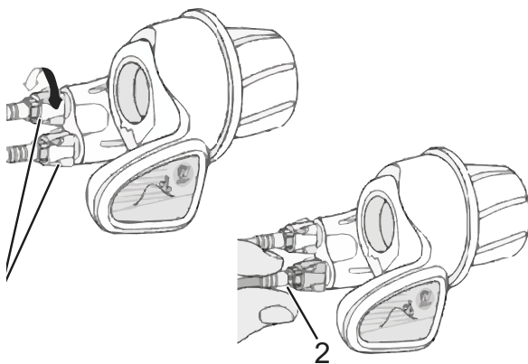
Figura 156: Puño giratorio con casquillos de ajuste (1) con holgura de giro (2)
