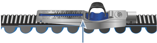
Figura 145: Calibre de comprobación en la correa
