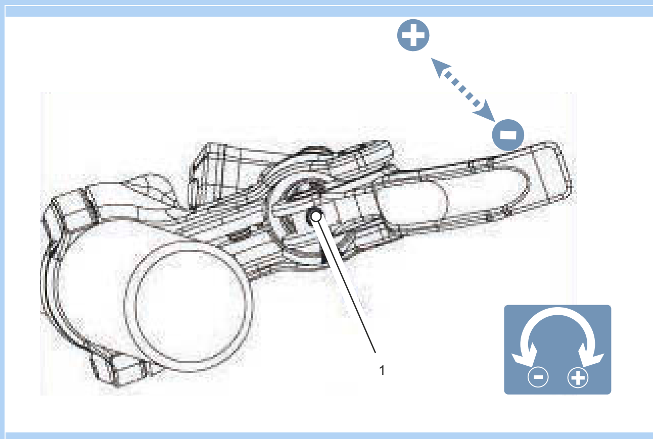
Figura 87: Posición del tornillo de ajuste (1)
