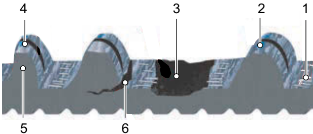
Figura 140: Signos de desgaste de una correa
