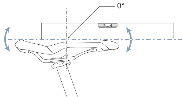
Figura 69: Inclinación del sillín horizontal con 0° de inclinación en el centro del sillín
