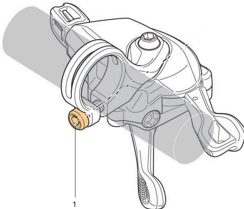
Figura 88: Posición del tornillo de fijación de la palanca de cambio SHIMANO (1)
