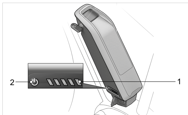
Figura 46: Posición del indicador de carga de la batería en el tubo del sillín
