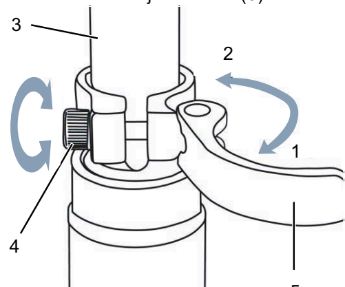
Figura 65: Apertura del cierre rápido de la tija de sillín
