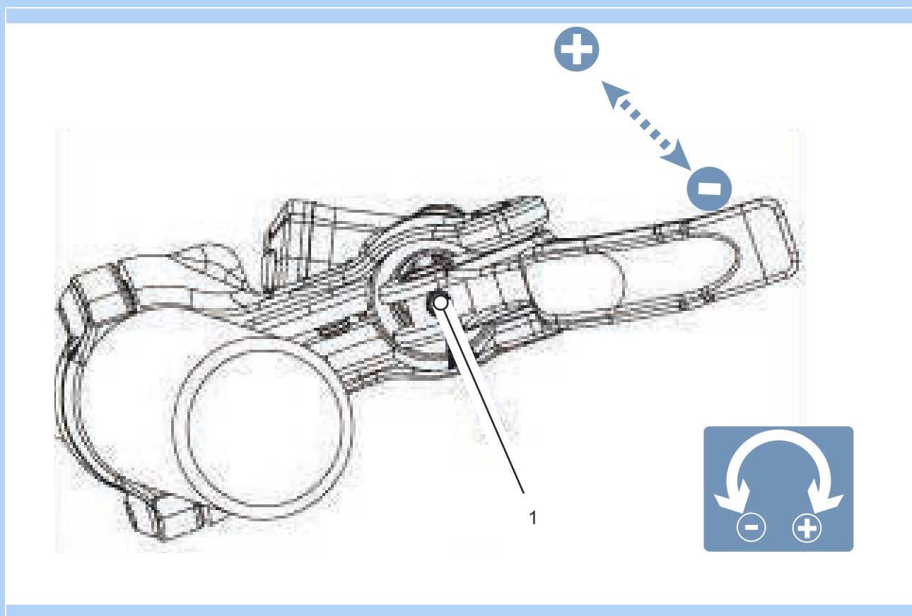
Illustration 103 : Position de la vis de réglage (1)
