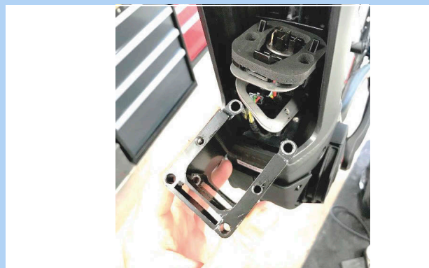
Illustration 55 : Retirer l'adaptateur PowerTube
