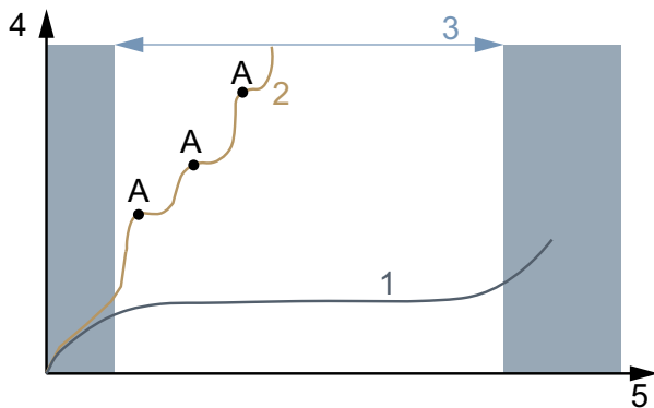
Illustration 157 : Diagramme d'usure, durée de service (x) par rapport à l'enlèvement de matière (y)
