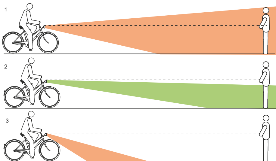
Illustration 105 : Feu réglé trop haut (1), correctement (2) et trop bas (3)
