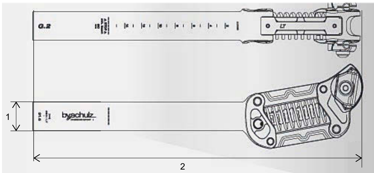
Illustration 50 : Dimensions de la tige de selle BY.SCHULZ, G2 avec diamètre (1) et longueur (2)
