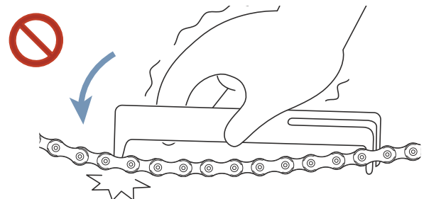
Illustration 173 : Le gabarit de mesure passe
