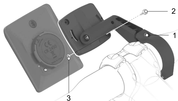
Illustration 112 : Position de la vis du jeu de direction
