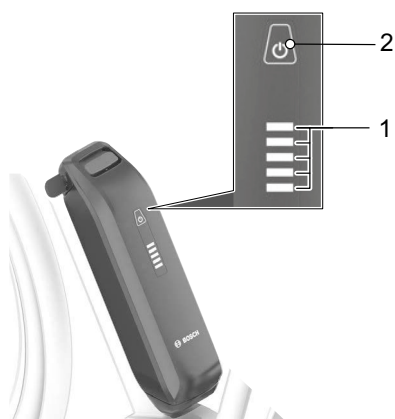
Illustration 45 : Éléments d'affichage et de commande de la batterie BOSCH PowerPack
