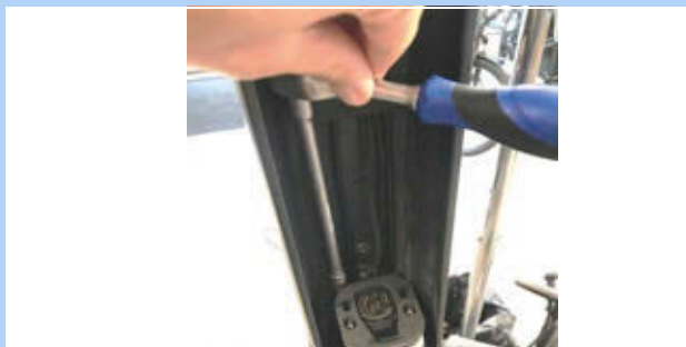
Illustration 54 : Retirer les vis à six pans creux
