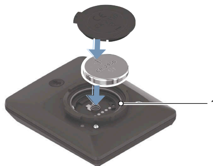
Illustration 109 : Insérer la pile en veillant à la position du joint (1)
