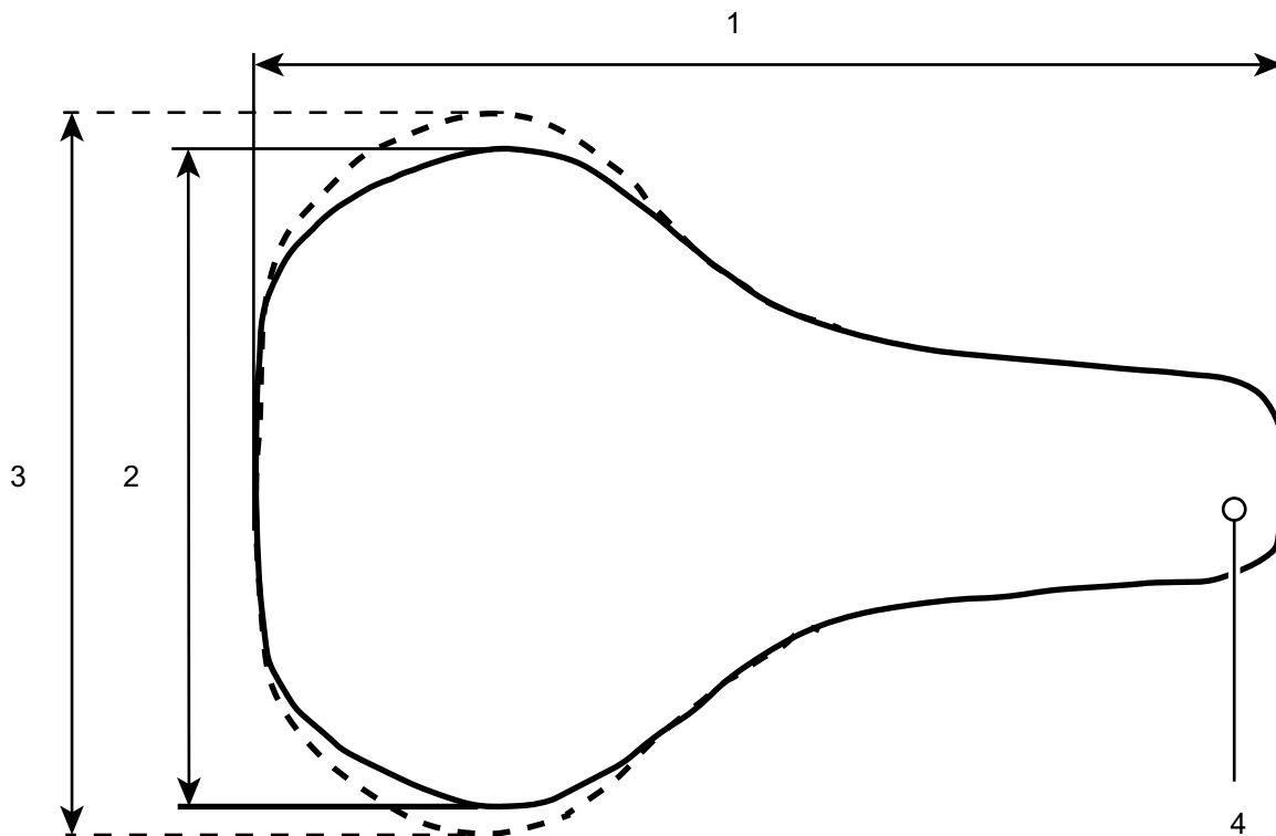
Illustration 19 : Dimensions de la selle
