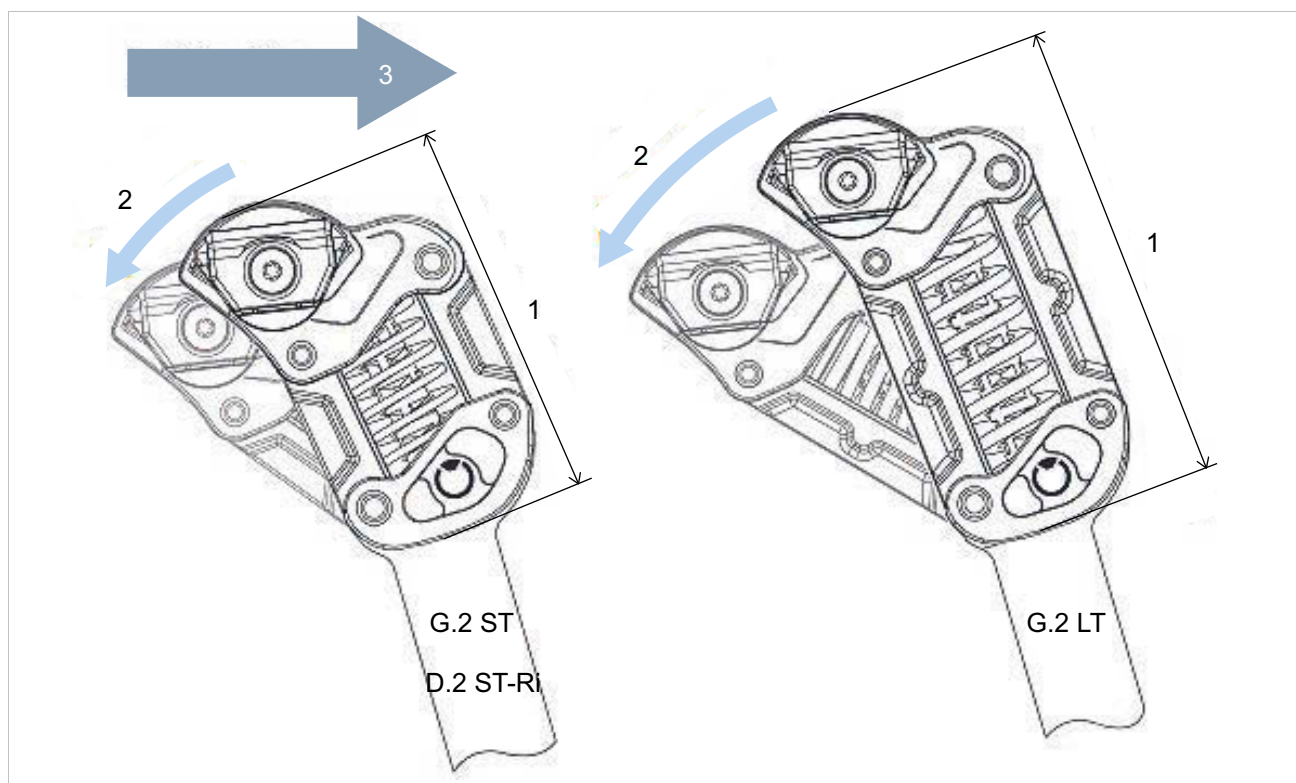
Illustration 49 : Caractéristiques techniques et fonctions des G.2 ST et G.2 LT avec hauteur de montage (1) et profondeur d'enfoncement à l'arrière (2) dans le sens de la marche (3)
