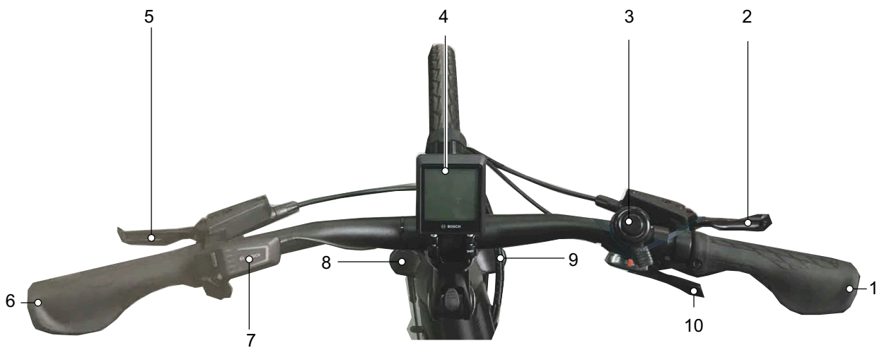
Illustration 39 : Vue détaillée d'un guidon avec BOSCH Kiox300, exemple
