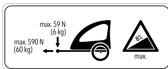
Illustration 115 : Plaque d'information de la remorque
