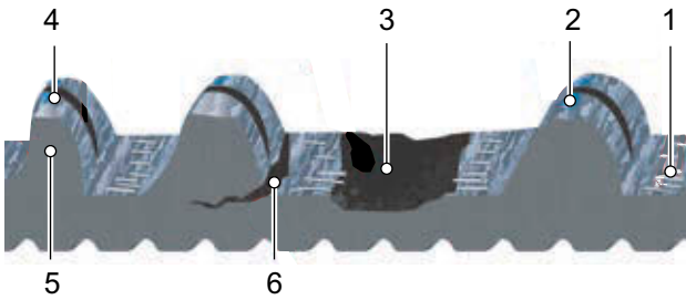
Illustration 174 : Signes d'usure d'une courroie
