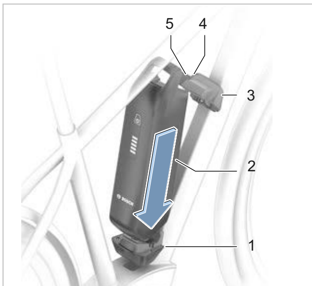
Illustration 135 : Insérer la batterie PowerPack
