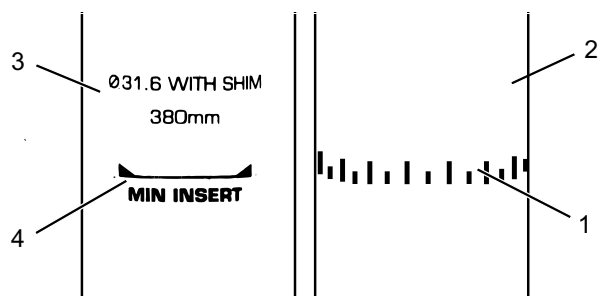
Illustration 82 : Vue détaillée de la tige de selle, exemples de marquage de la profondeur d'insertion minimale
