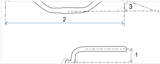
Illustration 7 : Dimensions du guidon
