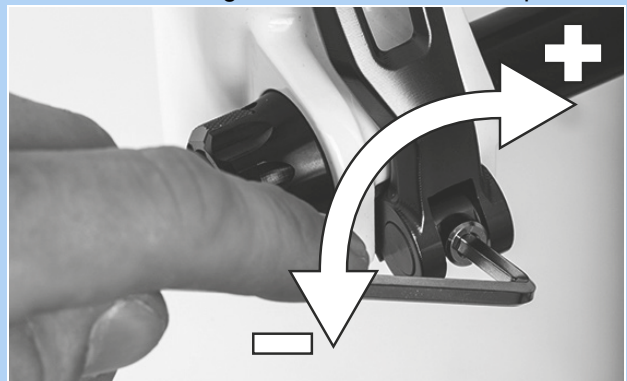
Illustration 192 : Régler la force de serrage de l'attache rapide
