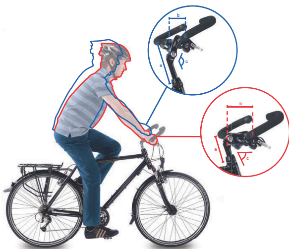
Illustration 93 : Position sur vélo de ville (en bleu) et sur vélo tout chemin (en rouge) avec modification de l'angle
