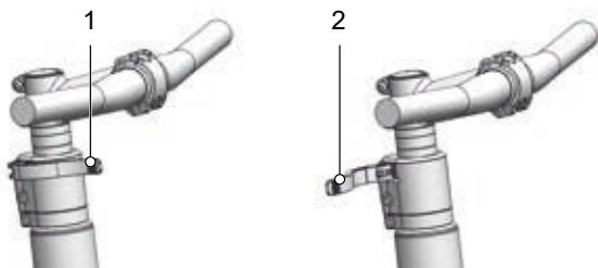
Illustration 88 : Levier de serrage de la potence fermé (1) et ouvert (2), exemple d'un All Up
