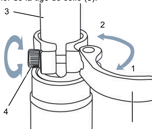
Illustration 81 : Ouvrir l'attache rapide de la tige de selle
