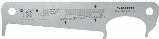
Illustration 167 : Exemple d'un gabarit de mesure SRAM
