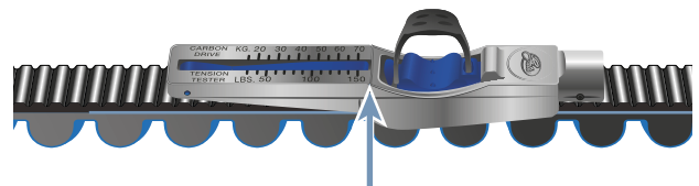
Illustration 179 : Gabarit de contrôle sur la courroie
