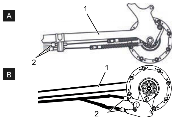
Illustration 189 : Douilles de réglage (2) sur deux modèles alternatifs (A et B) d'un changement de vitesse actionné par câble à deux câbles sur la base de cadre (1)
