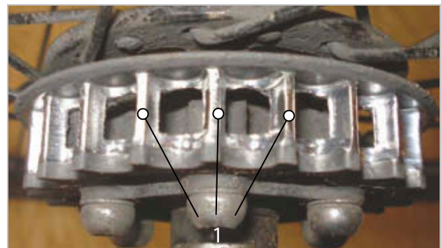
Figur 158: Foto med eksempel på slidt tandprofil
