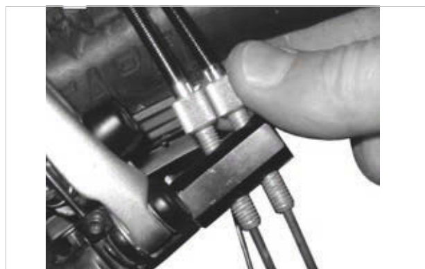
Figur 168: På udgaver af ROHLOFF-nav med intern skifteaktivering sidder kabelindstilleren på kabelmodholdet
