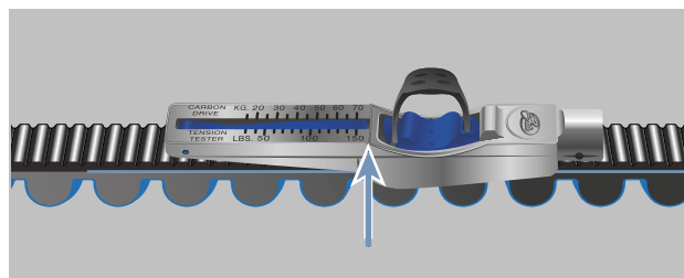
Figur 160: Kontrollære på rem
