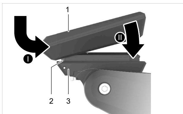
Figur 95: Isætning af displayet
