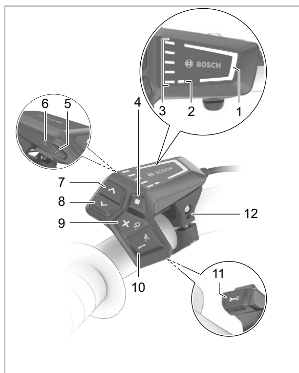
Figur 124: Oversigt over cykelcomputeren BOSCH LED Remote
