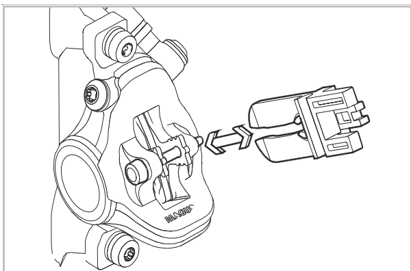
Figur 51: Fastgørelse af transportsikring
