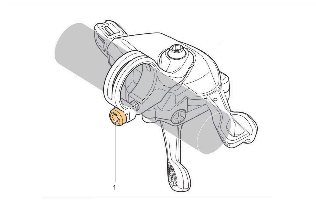
Figur 90: Monteringskruens position på SHIMANO-gearvælger (1)
