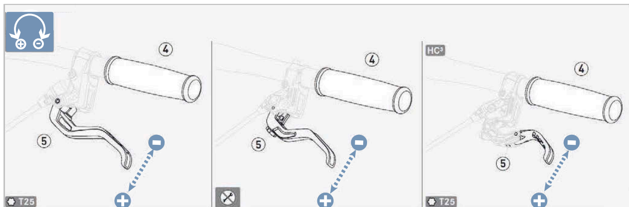
Figur 87: Indstilling af håndbremsens grebsbredde på MAGURA-skivebremse
