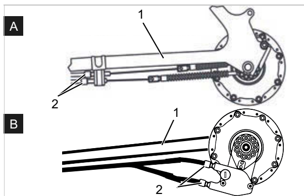
Figur 170: Slutmuffer (2) på to alternative udførelser (A og B) af et gearskifte med to kabler på baggaflen (1)
