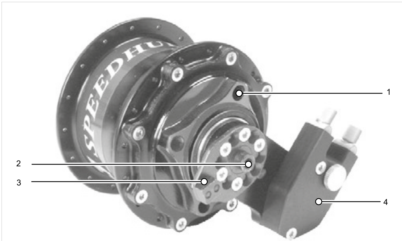
Figur 49: Tekniske data og funktioner for ROHLOFF, Speedhub 500/14 CC DB OEM, black, 32 holes, med skivebremsedæksel (1), hurtigbæspændingsaksel (2), CC OEM arbejdsplade (3) og ekstern skifteaktivering (4)
