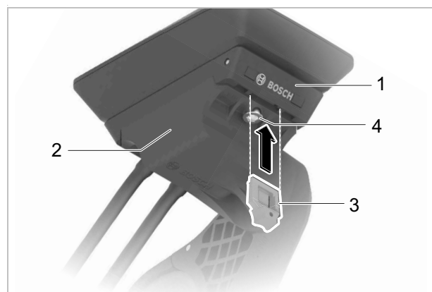
Figur 96: Styresætskruens position
