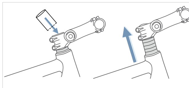
Figur 77: Forhøjning af Ahead-frempind ved at montere afstandsringe (spacers)
