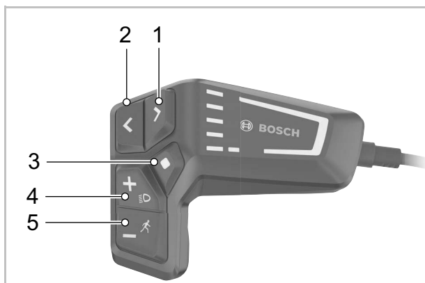
Figur 98: Betjeningselementer på BOSCH LED Remote
