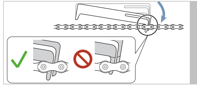
Figur 151: Målelæren sættes i
