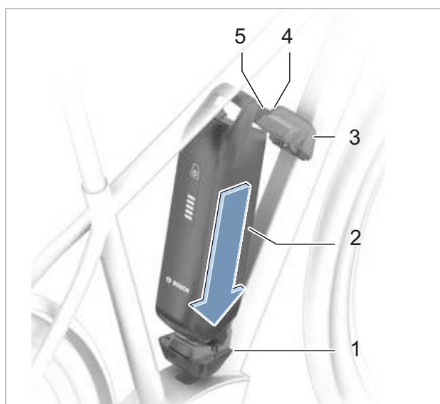
Figur 121: Isætning af PowerPack-batteri
