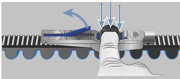
Figur 161: Tryk kontrollæren ned med fingeren
