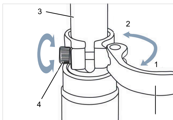
Figur 67: Løsning af sadelpindens hurtigbespænding
