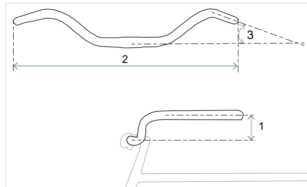
Figur 7: Styrets mål
