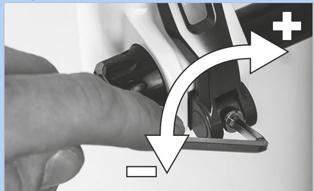
Figur 173: Indstilling af hurtigbespændingens spændekraft
