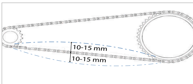
Figur 145: Eksempel på kontrol af kædestramning: 5 mm opad, 10 mm nedad = 15 mm afvigelse
