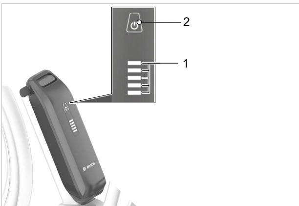
Figur 46: Indikator og betjeningsselement på BOSCH PowerPack-batteri
