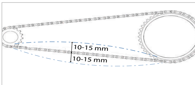
Figur 167: Eksempel på kontrol af kædestramning: 5 mm opad, 10 mm nedad = 15 mm afvigelse
