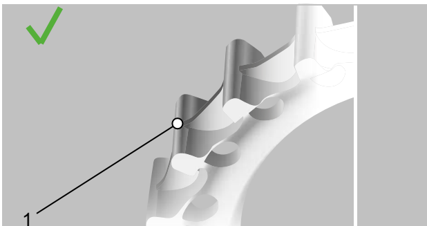
Figur 156: Optimal tandprofil
