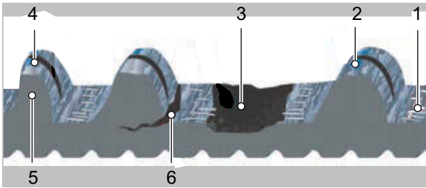
Figur 155: Tegn på slitage på en rem
