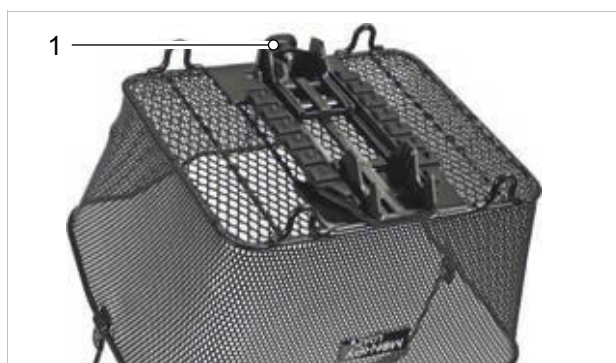
Figur 101: Kurv med MonkeyLoad-adapterplade og trækknop (1)
