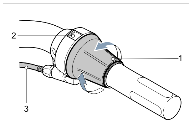
Figur 132: Gearskifte SHIMANO SL-C30000-70
