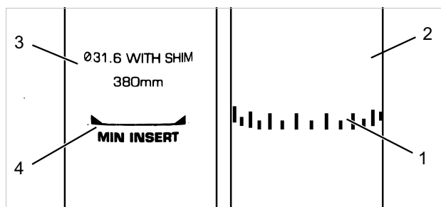
Figur 68: Detaljeret visning af sadelpind, eksempler på markering af minimumsdybden
