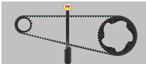
Figur 163: Ophængt målestang
