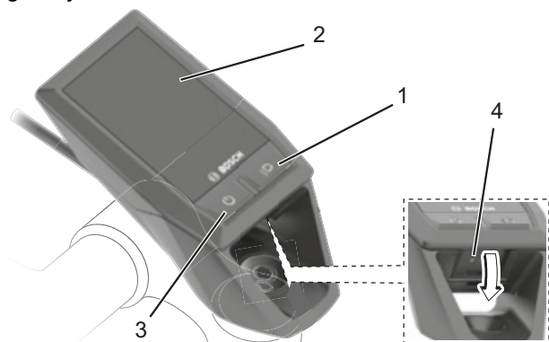
27. ábra: BOSCH Kiox fedélzeti számítógép felépítése
