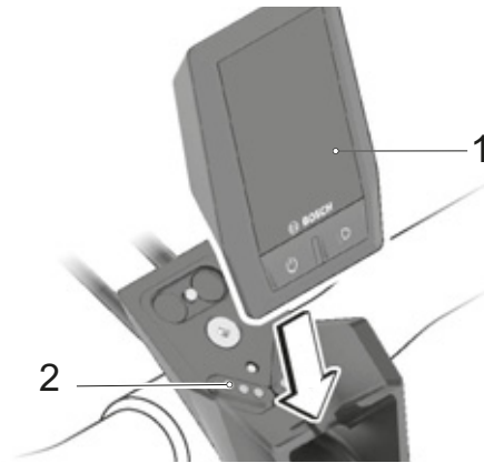
70. ábra: A fedélzeti számítógép (1) behelyezése
