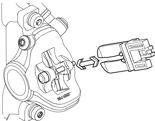
36. ábra: Szállítási rögzítés megfogatása
