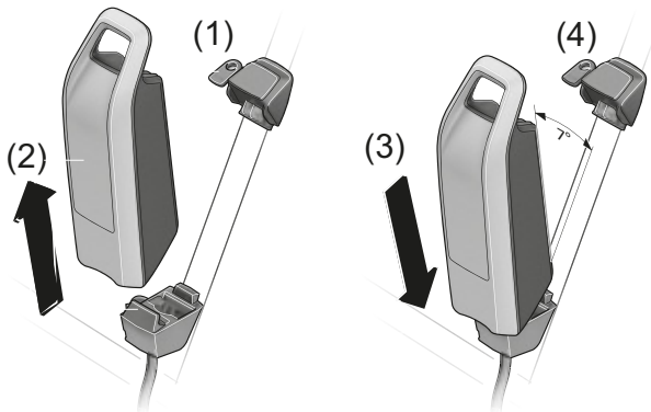
83. ábra: Vázakkumulátor kiserelése és beszerelése
