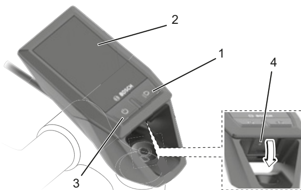
69. ábra: A fedélzeti számítógép felépítésének és kezelőszerveinek áttekintése
