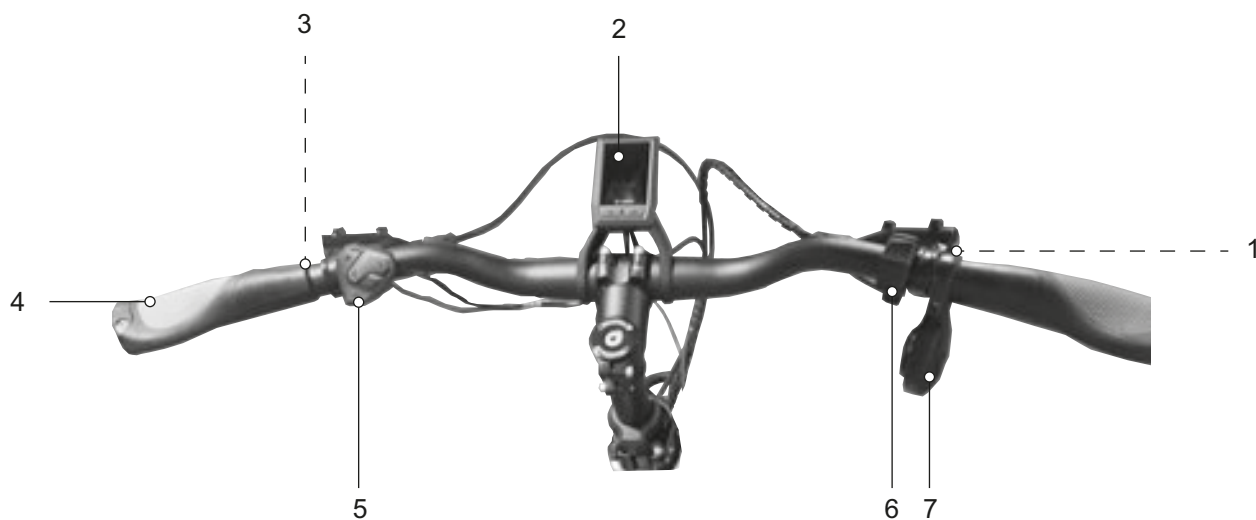
26. ábra: BOSCH Kiox fedélzeti számítógéppel felszerelt kormány részletes nézete, példa
