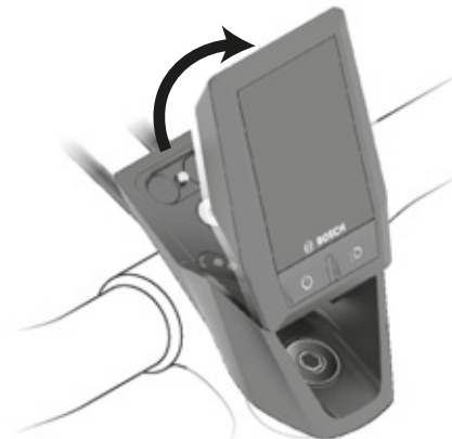
73. ábra: A fedélzeti számítógép levétele
