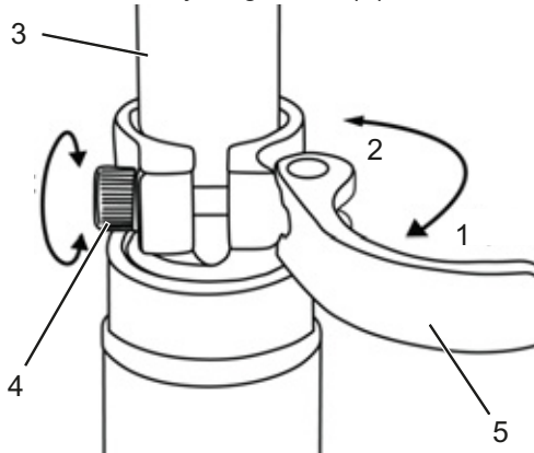
46. ábra: A nyeregcső gyorszárjának nyitása
