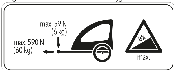
Afbeelding 76: Waarschuwingsticker aanhanger
