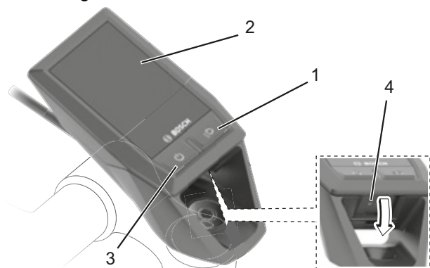
Afbeelding 27: Opbouw BOSCH Kiox boordcomputer
