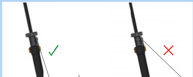
Afbeelding 117: Stand bowdenkabel
