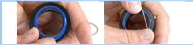
Afbeelding 160: Afstrijker inleggen en bevestigen
