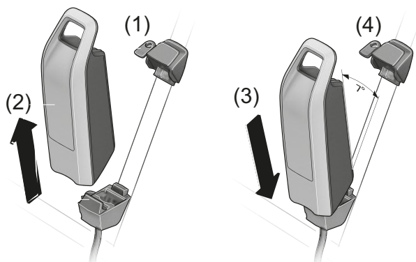
Afbeelding 83: Frame-accu verwijderen en aanbrengen
