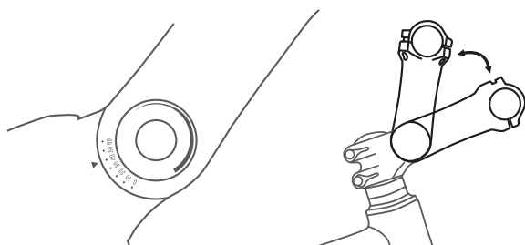
Afbeelding 57: Verschillende versies van in hoek verstelbare voorbouwen
