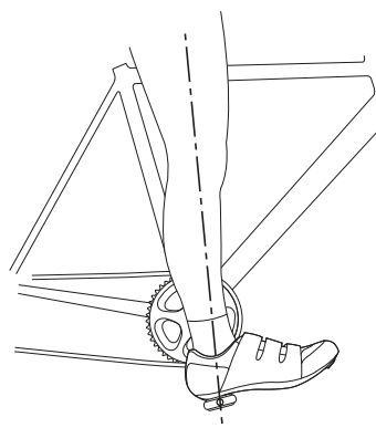
Afbeelding 45: Hielmethode
