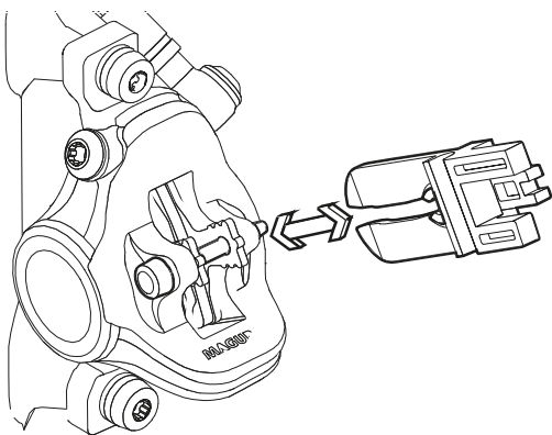
Afbeelding 36: Transportbeveiliging bevestigen
