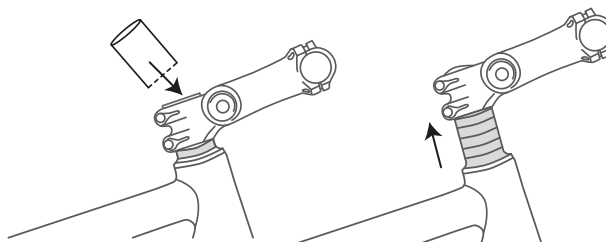
Afbeelding 56: Ahead voorbouw door montage van afstandsringen (spacers) verhogen
