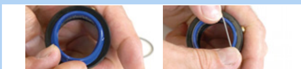
Figura 129: Inserción y fijación del rascador
