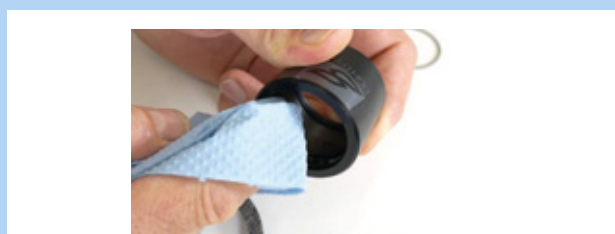
Figura 127: Limpieza del manguito exterior
