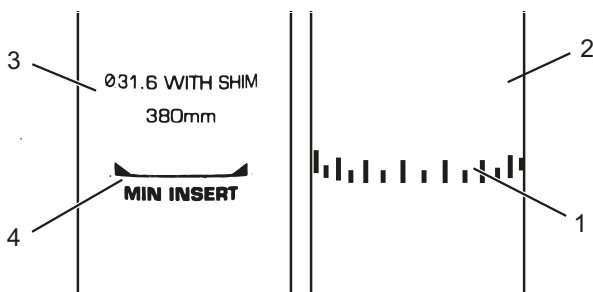
Figura 52: Vista detallada de las tijas de sillín, ejemplos de las marcas de la profundidad de inserción mínima
