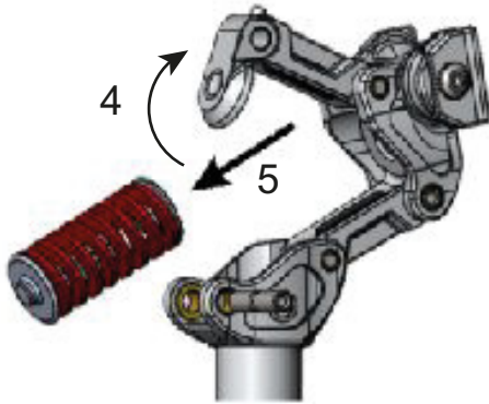
Figura 58: Giro el brazo de suspensión hacia atrás (4) y extracción del elemento de suspensión
