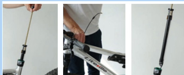
Figura 119: Extracción del cartucho
