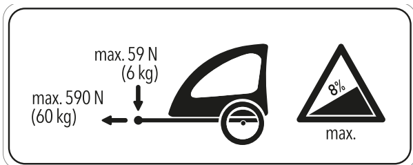
Figura 82: Placa indicadora de remolque
