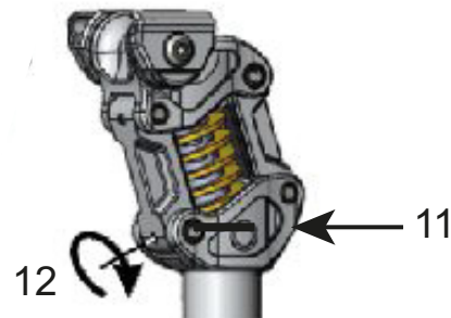
Figura 61: Engrase del eje de acero inoxidable (11) y apriete del tornillo prisionero de fijación M5
