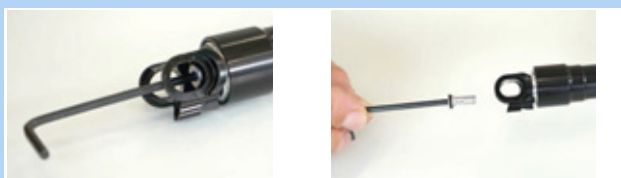
Figura 135: Desenroscar la tapa de la válvula
