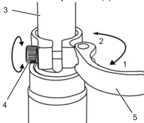
Figura 51: Apertura del cierre rápido de la tija de sillín
