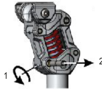
Figura 56: Desenroscado del tornillo prisionero (1) y extracción del eje de acero inoxidable (2)
