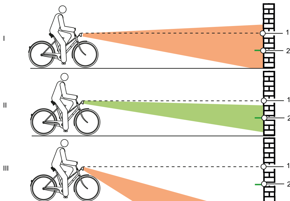
Figura 105: Luz ajustada demasiado alta (1), correctamente (2) y demasiado baja (3)
