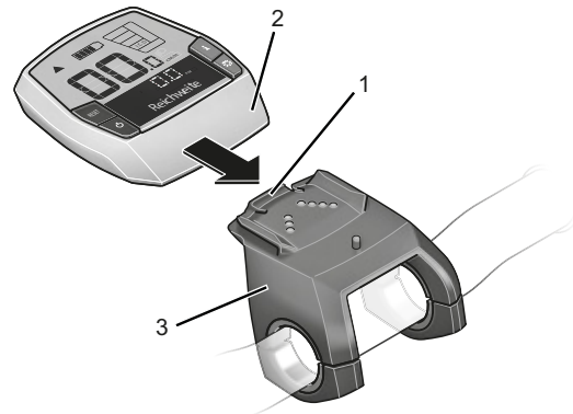
Figura 81: Inserción del ordenador de a bordo (2) a través del tope móvil del ordenador de a bordo (1) hasta el tope del soporte (3)
