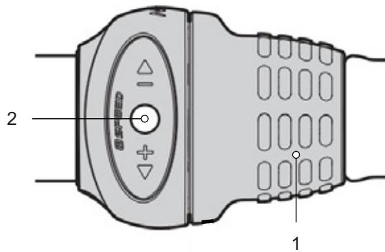
Figura 35: Cambio de marchas SHIMANO SL-C30000-7, vista desde arriba
