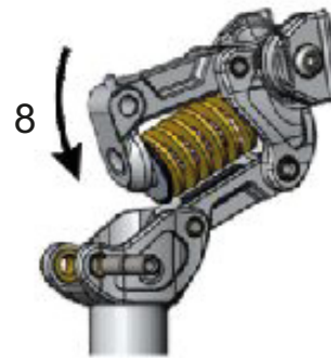
Figura 60: Giro del brazo de suspensión hacia delante (8)
