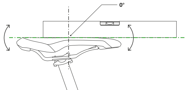
Figura 55: Inclinación del sillín horizontal con 0° de inclinación en el centro del sillín
