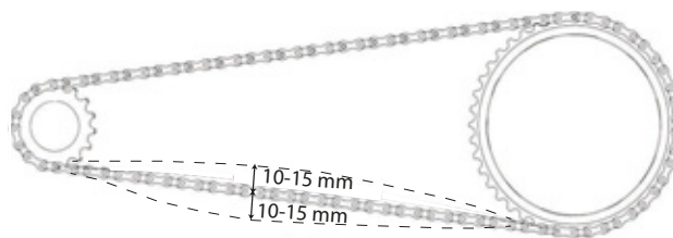
Figura 106: Comprobación de la tensión de la cadena
