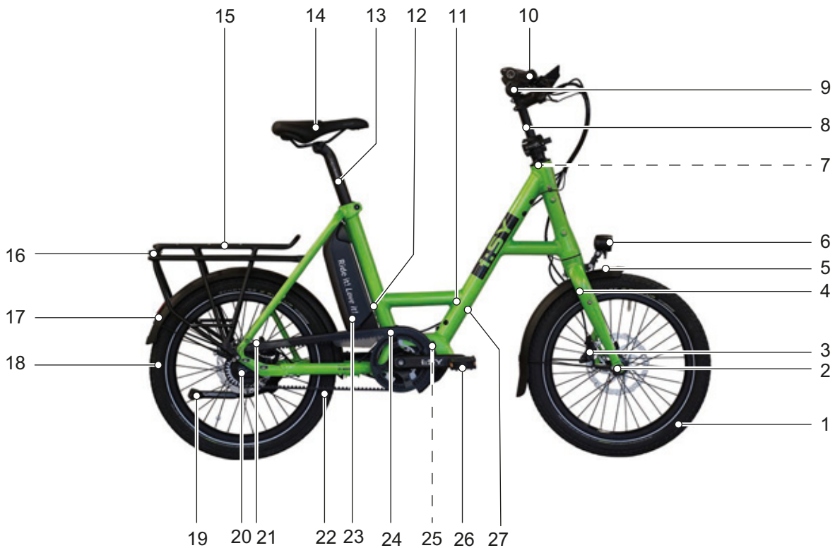
Figura 2: Pedelec visto desde el lado derecho
