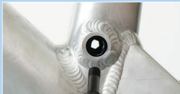
Figura 175: Orificio de la interfaz Postpin
