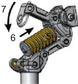
Figura 59: Colocación del elemento de suspensión (6) y cierre del elemento de suspensión
