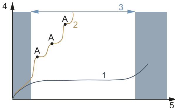
Figura 98: Diagrama de desgaste, vida útil (x) con respecto a desgaste de materiales (y)
