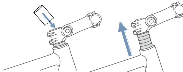
Illustration 75 : Relever la potence Ahead en montant une rondelle d'écartement
