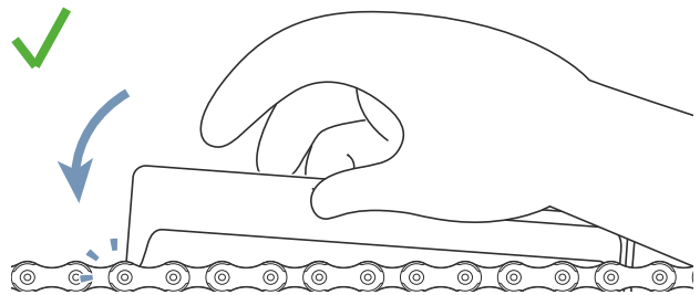
Illustration 138 : Le gabarit de mesure ne passe pas
