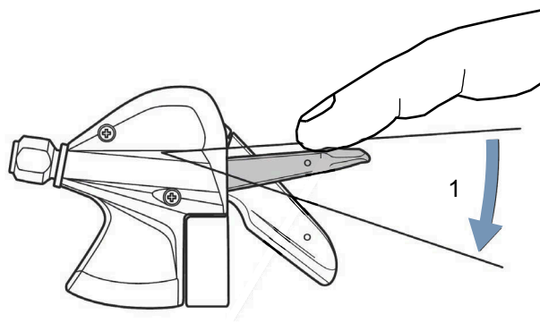
Illustration 117 : Changement de vitesse avec manette B, exemple d'un changement de vitesse SL-M315
