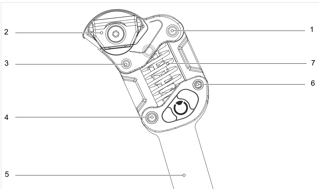
Illustration 25 : Structure de la tige de selle by.schulz G2
