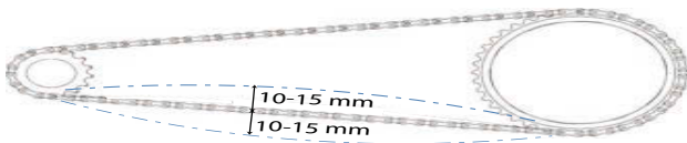
Illustration 130 : Exemple de contrôle de la tension de la chaîne : 5 mm vers le haut, 10 mm vers le bas = écart de 15 mm
