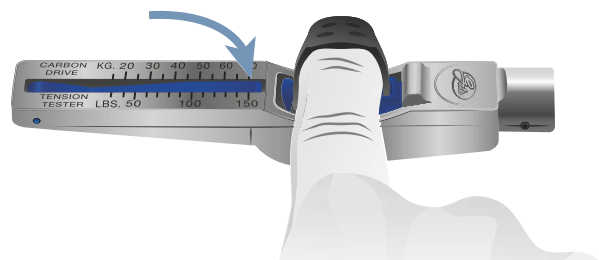
Illustration 144 : Index dans le gabarit de contrôle
