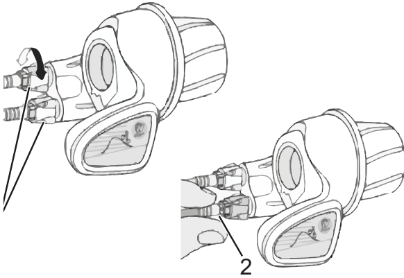
Illustration 156 : Poignée de vitesse rotative avec douilles de réglage (1) avec jeu de rotation (2)
