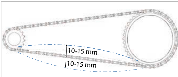
Illustration 152 : Contrôler la tension de la chaîne
