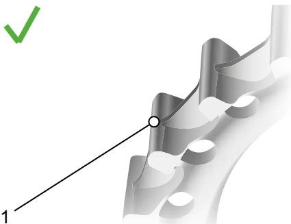
Illustration 141 : Profil de cran optimal
