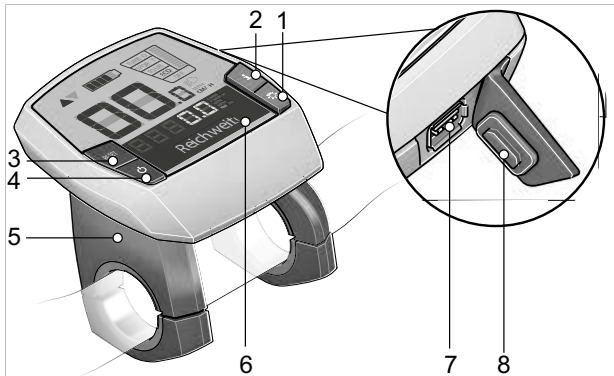
Illustration 39 : Structure de l'ordinateur de bord BOSCH Intuvia
