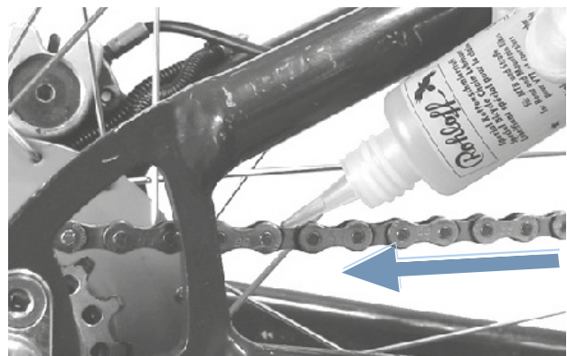
Illustration 124 : Lubrifier la chaîne
