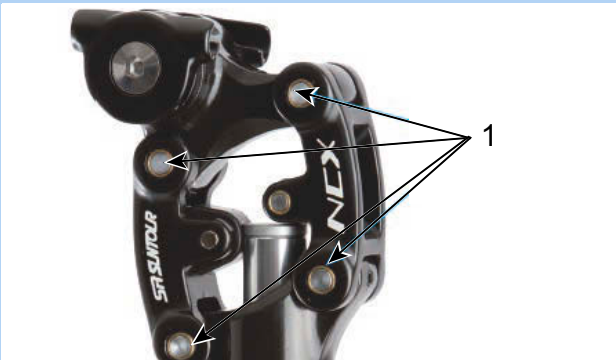
Illustration 159 : Points de lubrification de la tige de selle suspendue SR SUNTOUR
