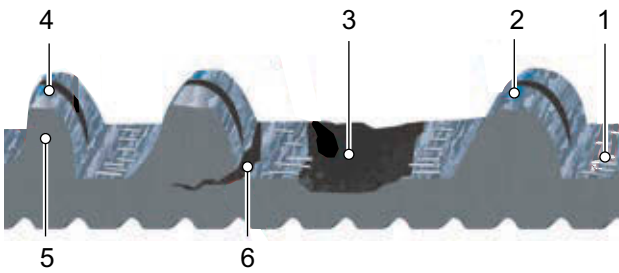
Illustration 140 : Signes d'usure d'une courroie
