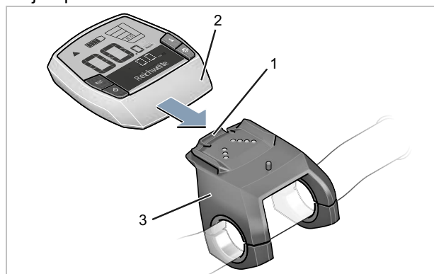
Illustration 92 : Enfoncez l'ordinateur de bord (2) via le dispositif de blocage de l'ordinateur de bord (1) jusqu'à la butée du support (3)
