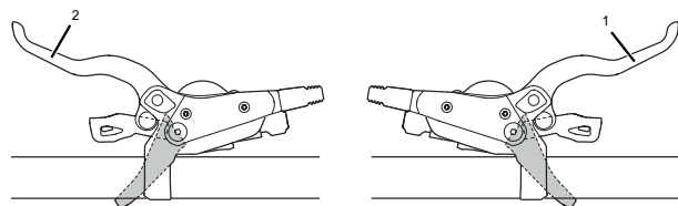
Illustration 115 : Frein à main arrière (1) et avant (2), exemple d'un frein SHIMANO
