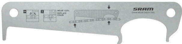
Illustration 133 : Exemple d'un gabarit de mesure SRAM
