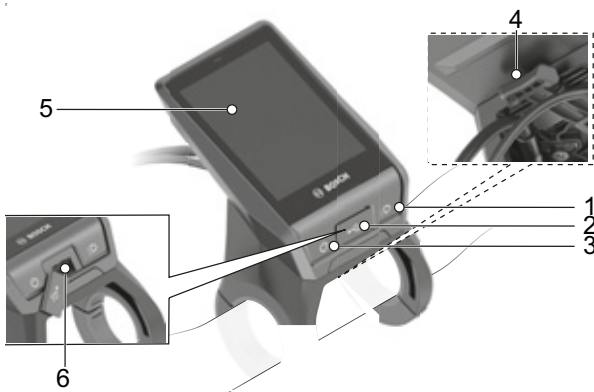
Illustration 26 : Structure de l'ordinateur de bord BOSCH Nyon
