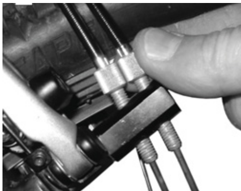
Illustration 120 : Sur les versions de moyeux ROHLOFF avec commande interne du changement de vitesse, le dispositif de réglage de la tension est situé sur le contre-support de tension.
