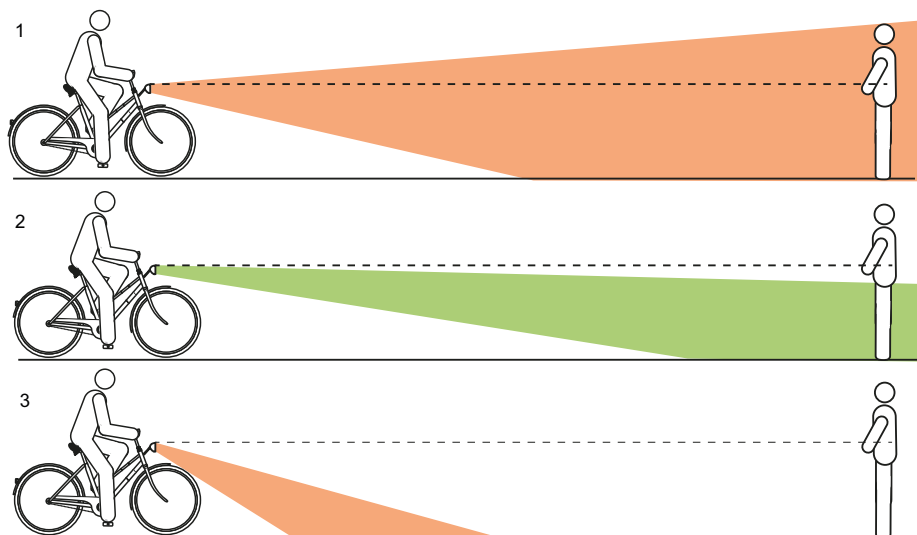
Illustration 73 : Feu réglé trop haut (1), correctement (2) et trop bas (3)
