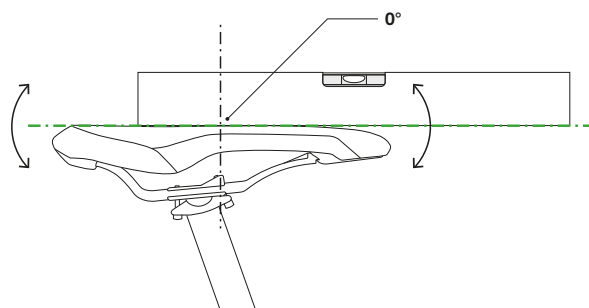
Illustration 57 : Inclinaison de la selle horizontale avec inclinaison de 0° au milieu de la selle
