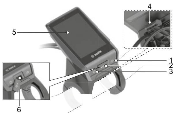
Illustration 76 : Aperçu de la structure et des éléments de commande de l'ordinateur de bord
